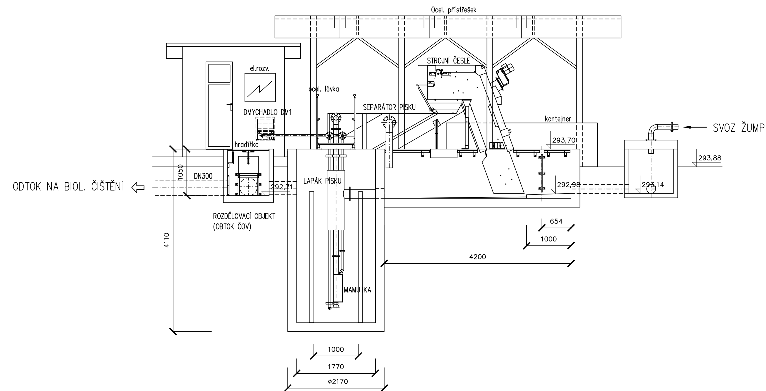
LEGENDA VIZ. TECHNOLOGICKÉ SCHÉMA ČOV
